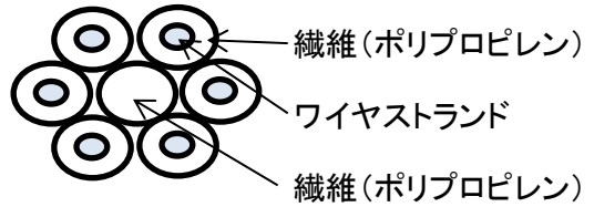
断面形状
